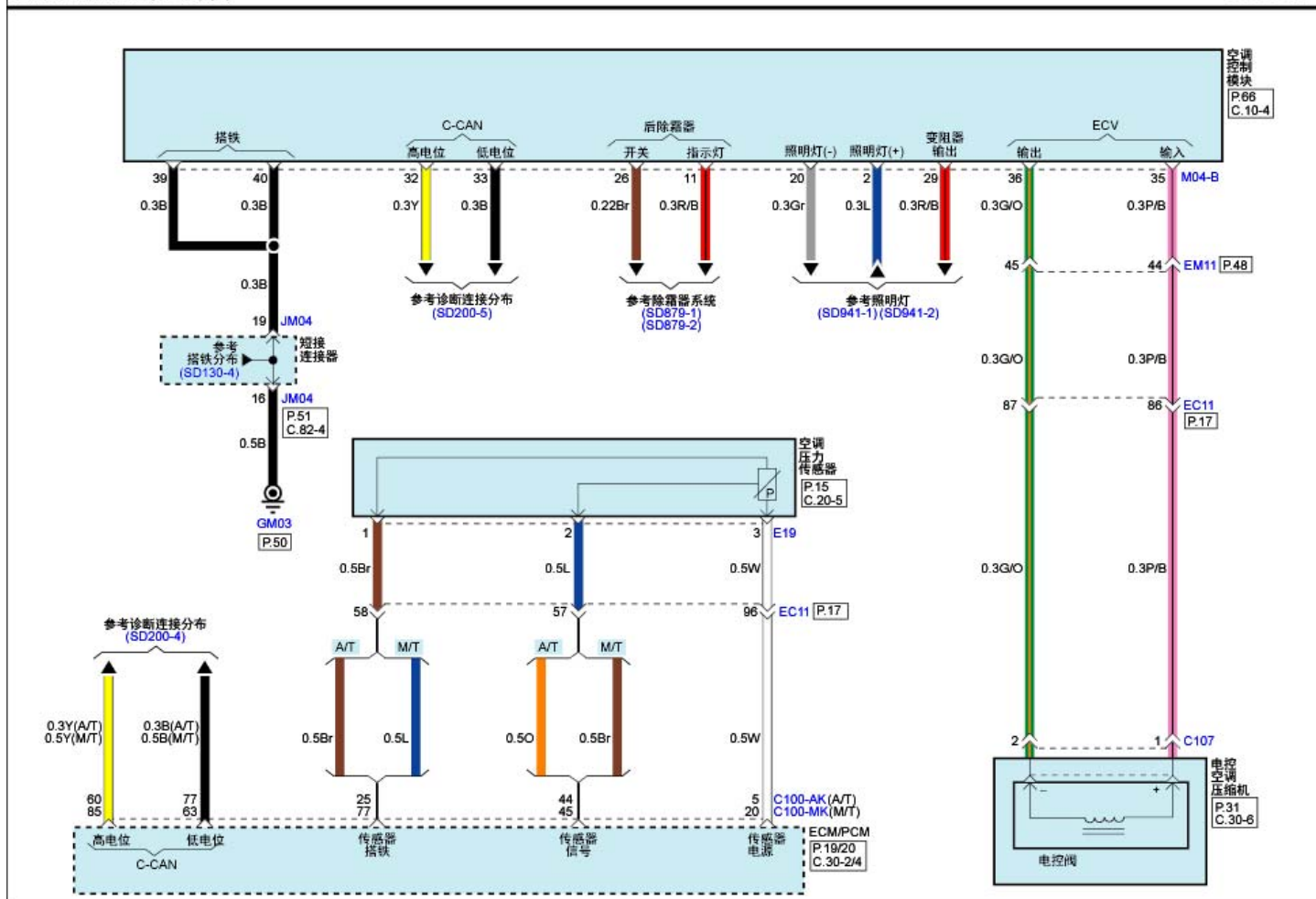
空调控制系统(手动)(3)
